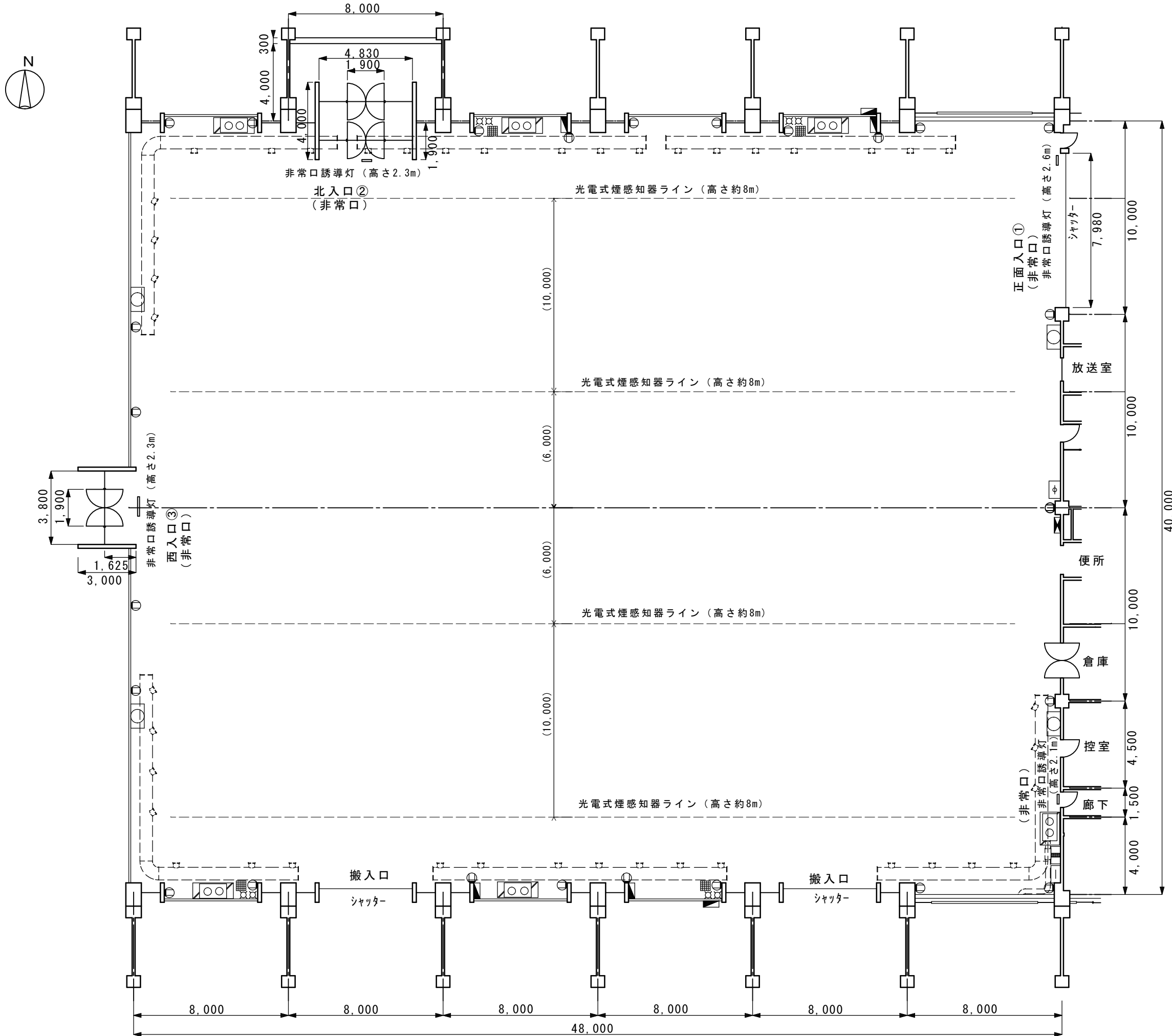
1階 第1展示場平面図 縮尺1:200
